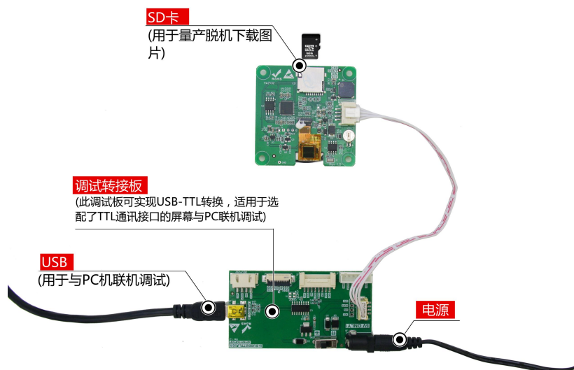
图 1-3 调试工具图
