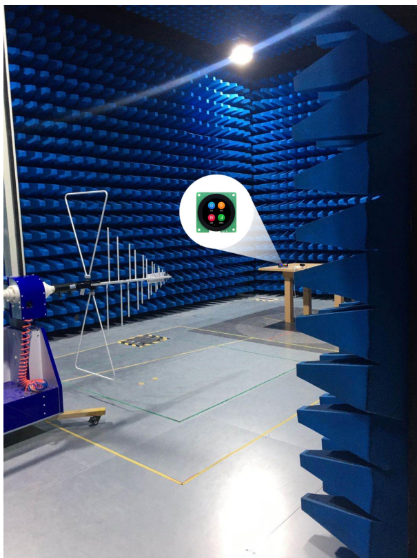
图 4-4 RE 测试图
