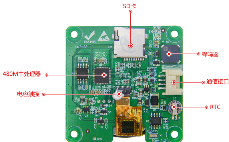
图 1-2 硬件配置图
