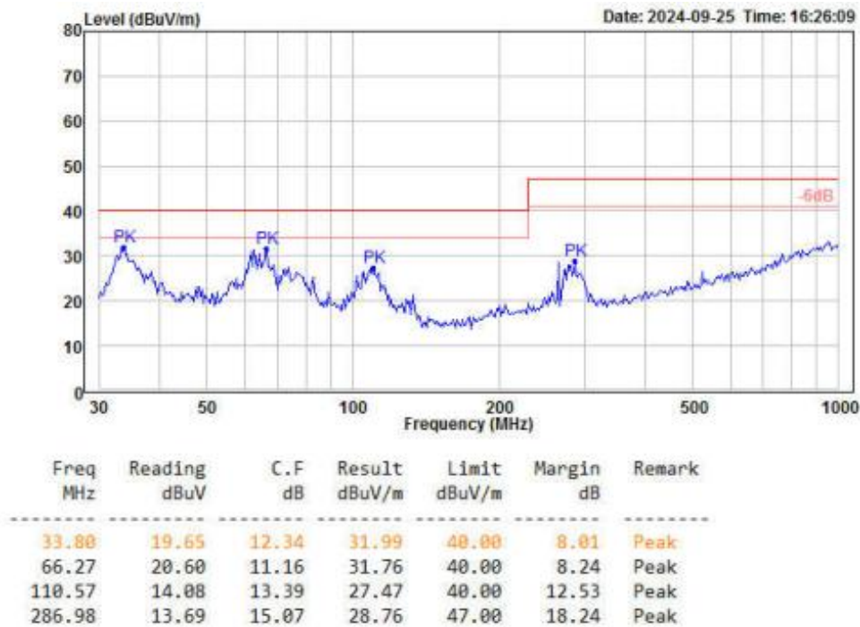
图 4-5 RE 测试水平方向
