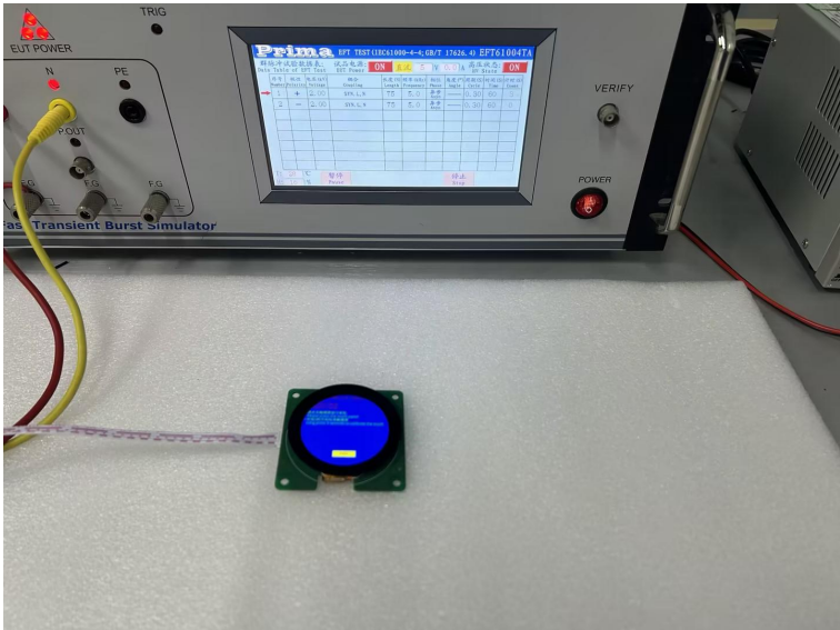
图 4-3 EFT 测试图
