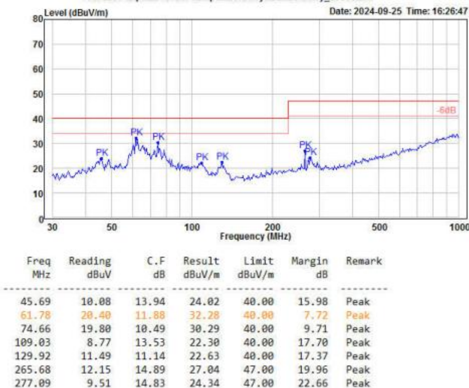
图 4-6 RE 测试垂直方向
