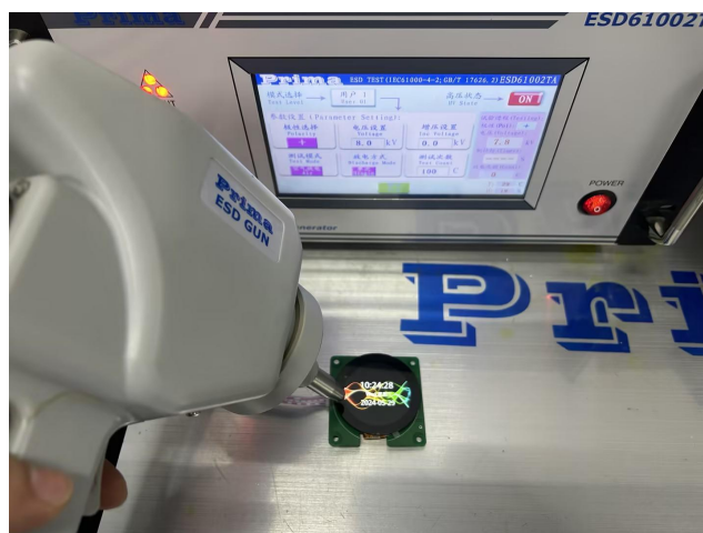
图 4-2 ESD 测试图
